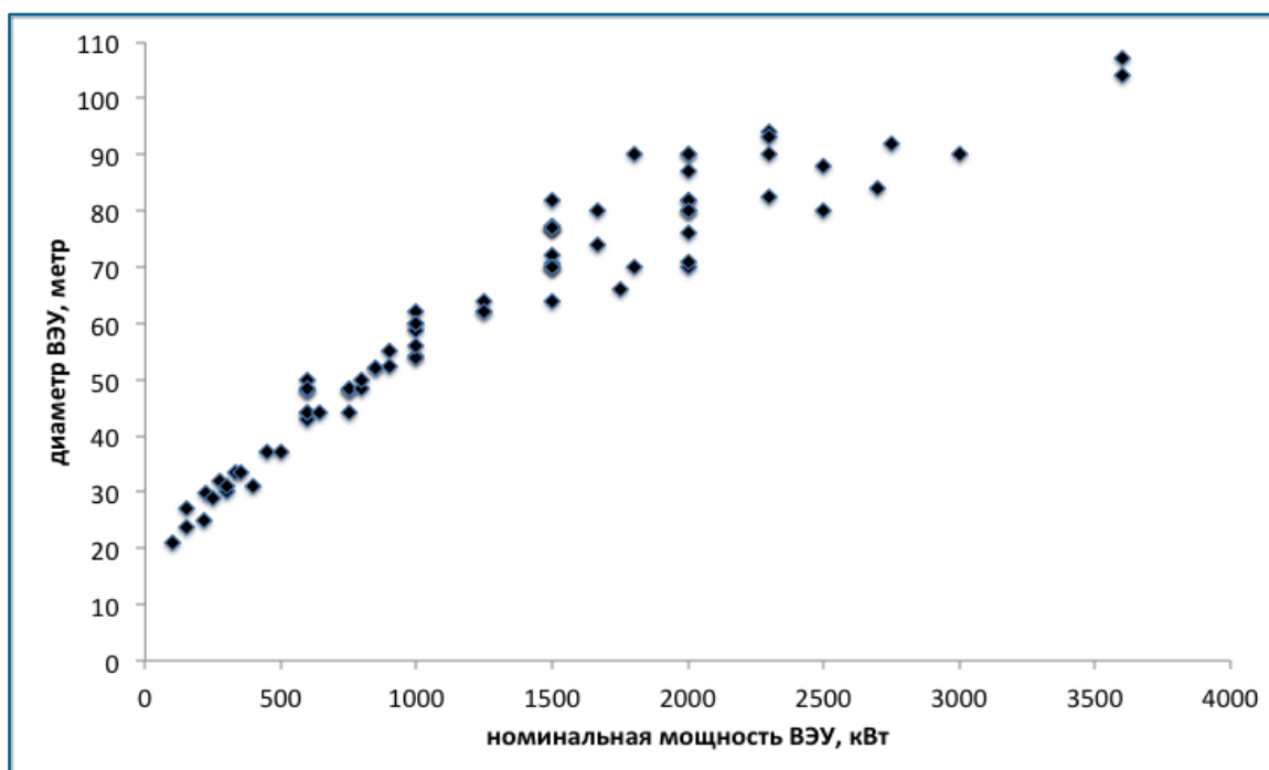
Рис. 58. Зависимость диаметра от номинальной мощности ВЭУ.
