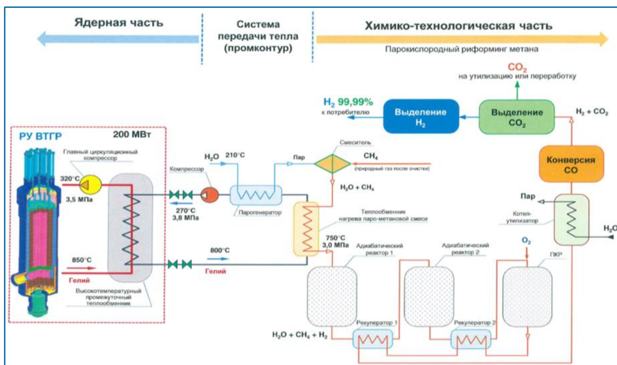
Рис. 99. Схема одного блока АЭТС с РУ ВТГР и ХТ [150]
