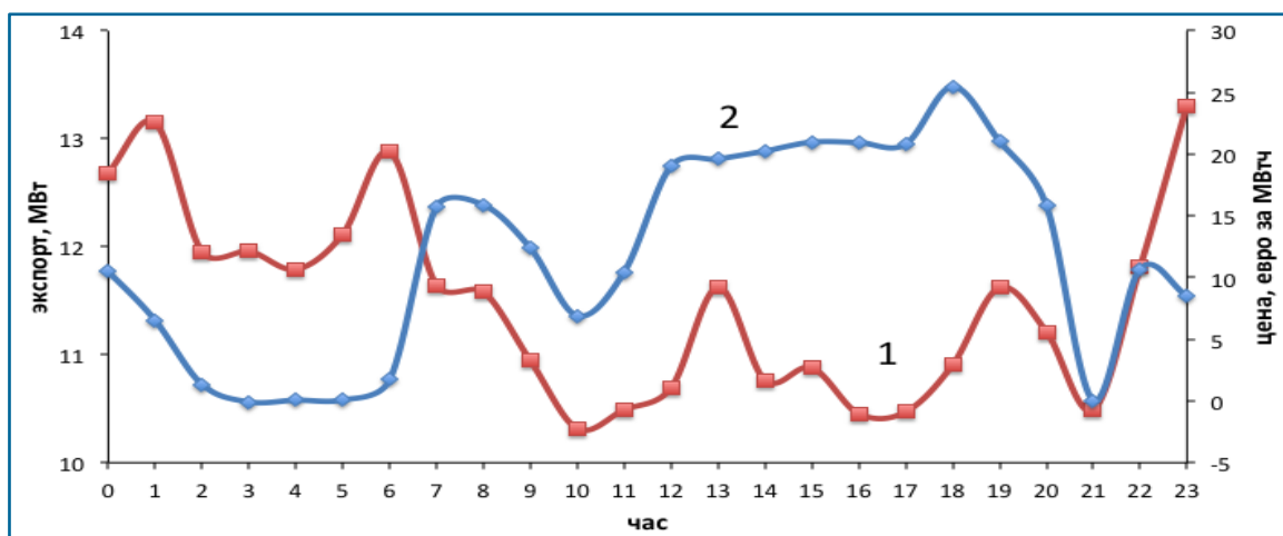
Рис. 54. Экспорт и цены 8 декабря 2018 года: 1 – экспорт электроэнергии из энергосистемы Германии; 2 – цена электроэнергии
