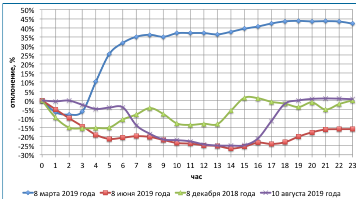
Рис. 16. Режимы загрузки энергоблоков АЭС в течение суток
