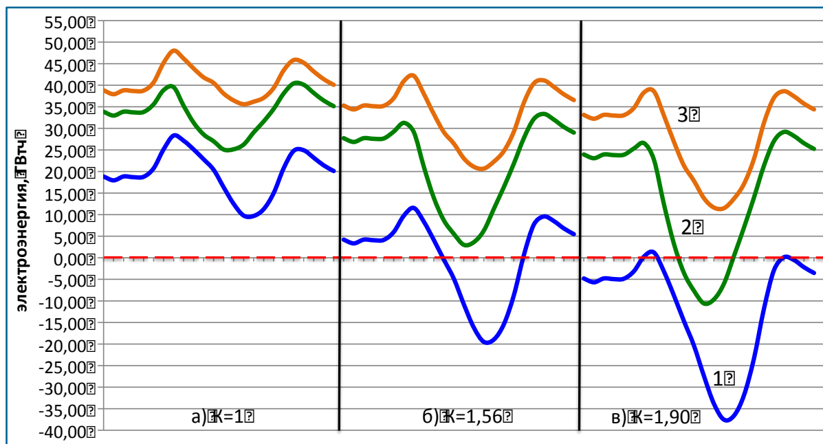
Рис. 29. График работы прочей генерации, включая ТЭС и АЭС, в июне: 1 – разница между потреблением электроэнергии и суточным максимумом выработки электроэнергии ВИЭ; 2 – разница между потреблением электроэнергии и среднесуточной выработкой электроэнергии ВИЭ; 3 – разница между потреблением электроэнергии и суточным минимумом выработки электроэнергии ВИЭ
