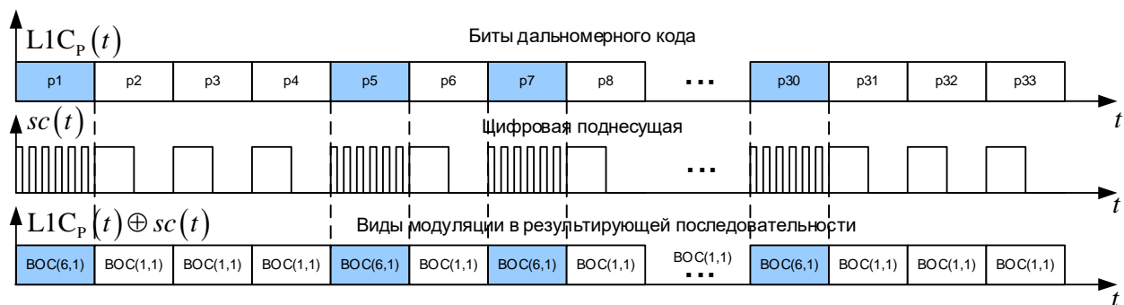
Рис. 4.4. Мультиплексная модуляция TMBOC(6,1,4/33) в радиосигнале GPS L1Cp
