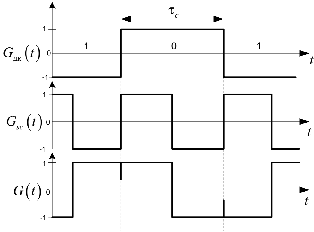
Рис. 2.3. Модуляция цифровой поднесущей
