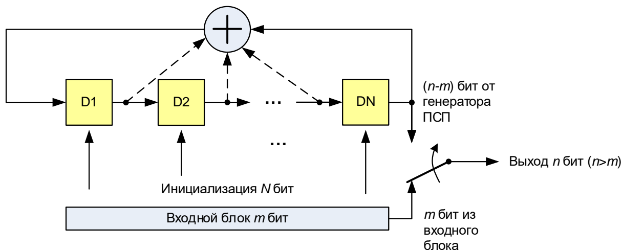
Рис. 5.4. Кодер БЧХ: VCH(n, m)
