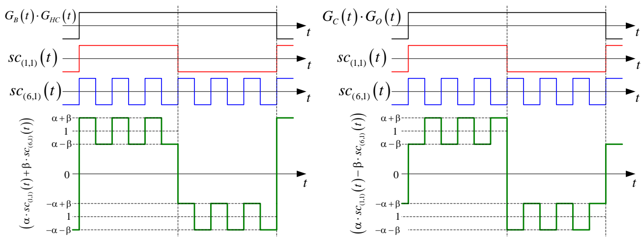
Рис. 4.5. Формирование составных модулирующих функций для сигнала с модуляцией СВОС
