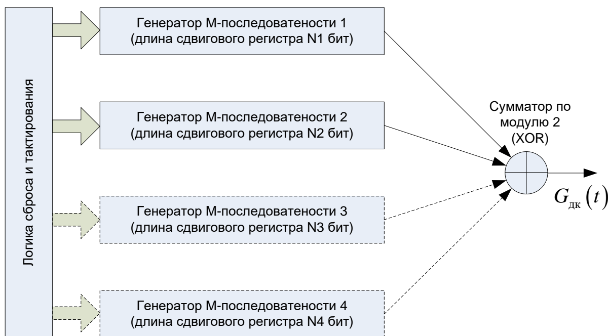
Рис. 3.3. Комбинирование М-последовательностей
