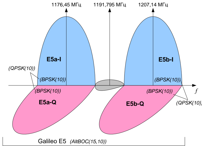
Рис. 4.6. Компоненты радиосигнала Galileo E5 с модуляцией AltBOC(15,10)
