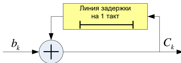
Рис. 5.2. ОФМ-кодер
