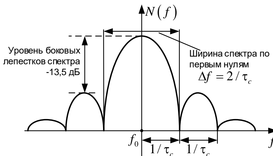
Рис. 2.2. Спектральная плотность мощности ФМ-2 радиосигнала
