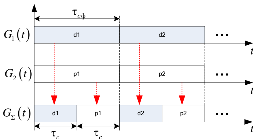
Рис. 4.2. Временное уплотнение сигналов
