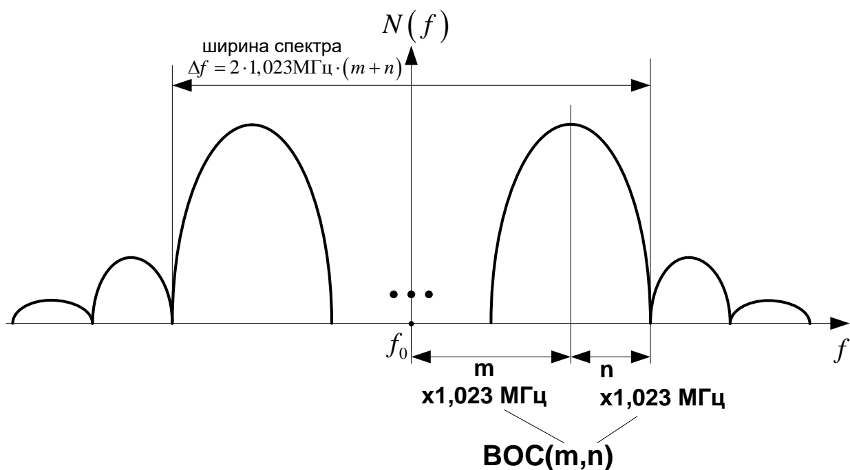
Рис. 2.4. Вид спектральной плотности мощности радиосигнала с ВОС модуляцией
