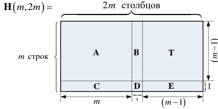
Рис. 5.5. Матрица проверок четности для LDPC-кодера
