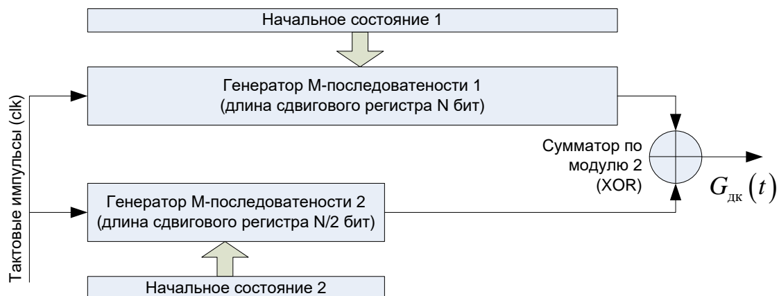
Рис. 3.5. Схема формирования кода Касами
