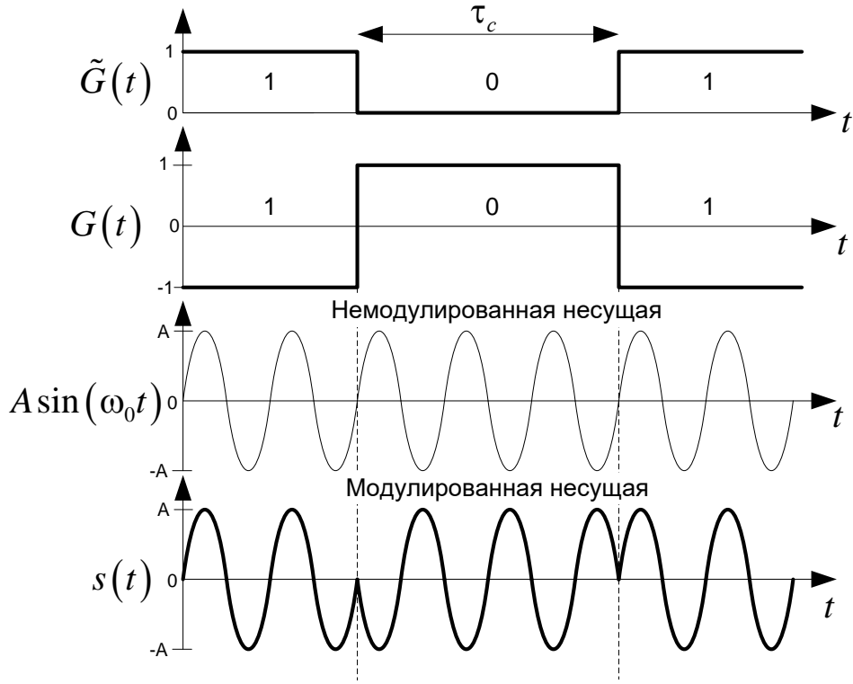
Рис. 2.1. Принцип бинарной фазовой манипуляции
