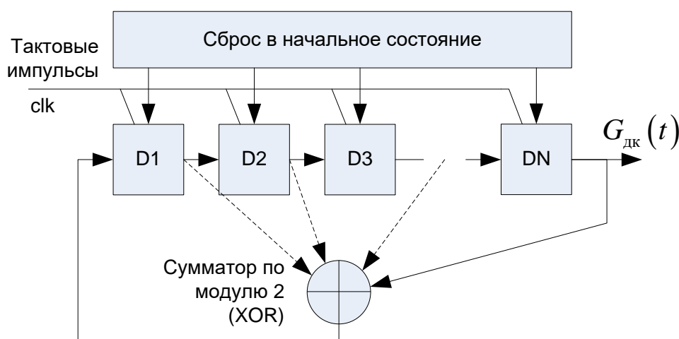
Рис. 3.2. Формирование М-последовательности
