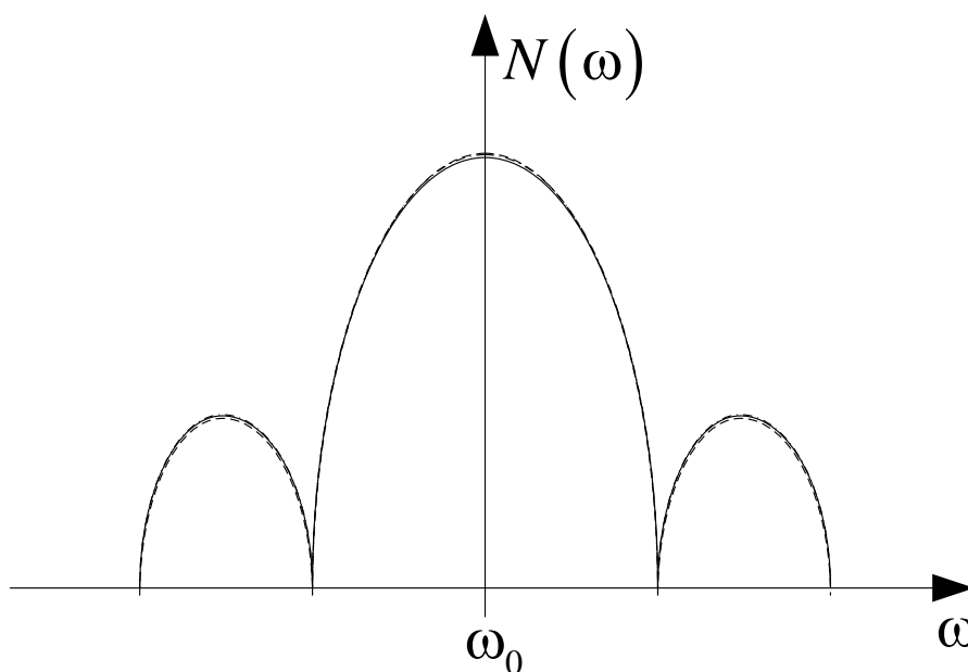
Рис. 1.1. График спектральной плотности мощности радиосигналов с кодовым разделением
