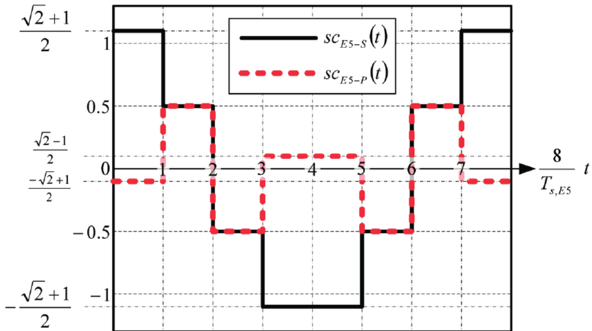
Рис. 4.7. Составные модулирующие функции для радиосигнала Galileo E5 с модуляцией AltBOC (показан один период)
