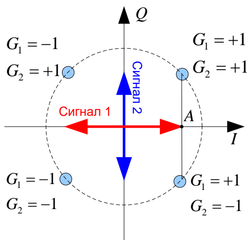
Рис. 4.1. Сигнальное созвездие при квадратурном уплотнении
