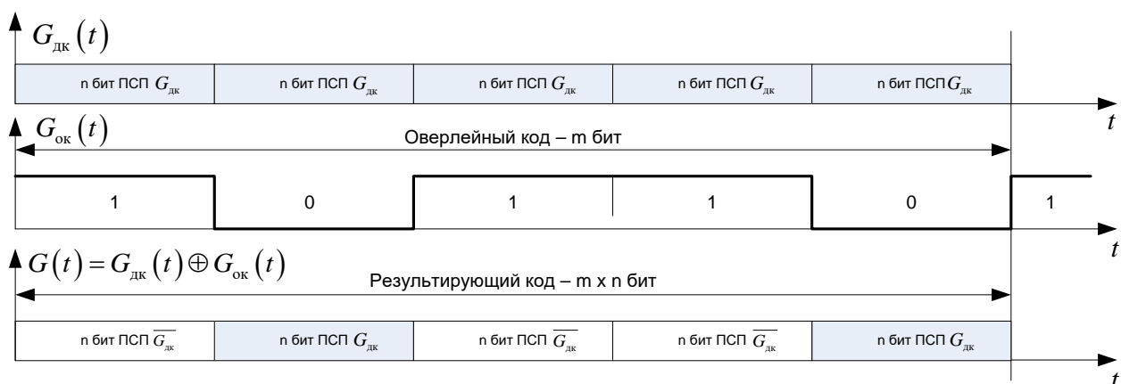
Рис.3.6. Наложение оверлейного кода
