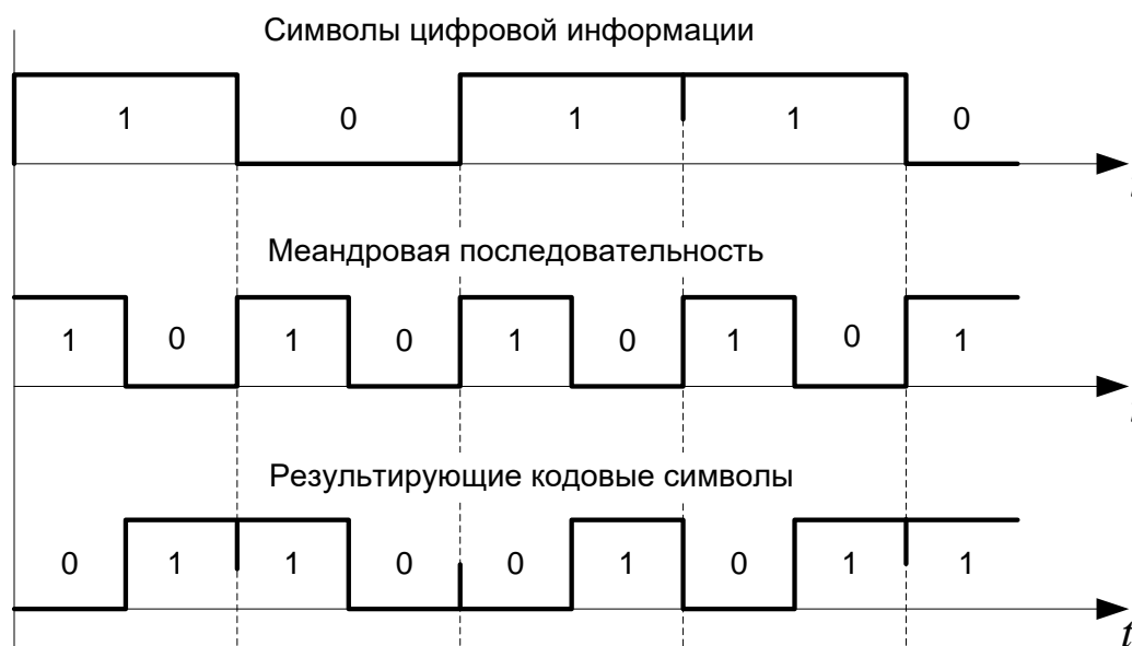
Рис. 5.1. Наложение меандра при кодировании навигационного сообщения
