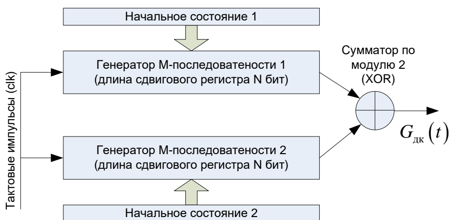
Рис. 3.4. Схема формирования кода Голда
