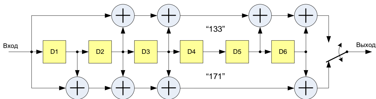
Рис. 5.3. Сверточный кодер FEC(133,171)
