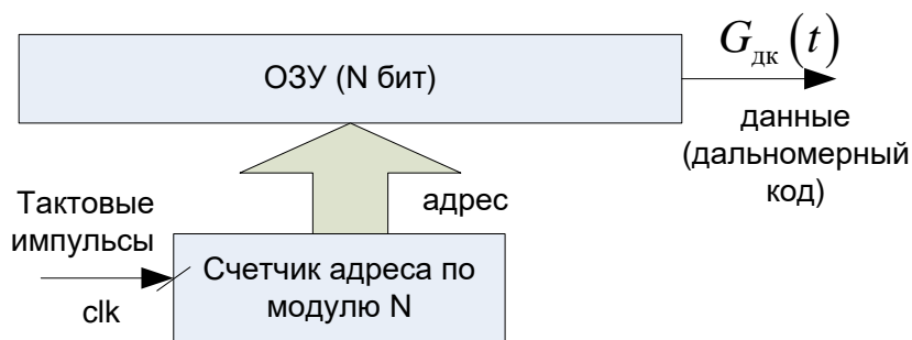
Рис. 3.1. Формирование дальномерного кода табличным методом
